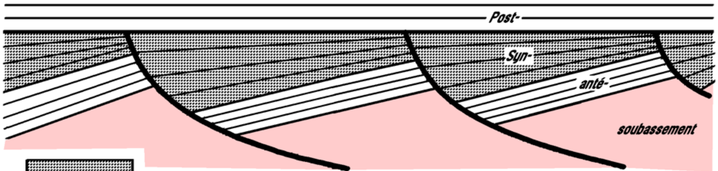
4 Failles synsédimentaires listriques ("blocs basculés")
