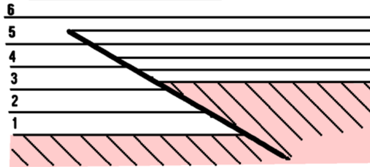
- b - Faille inverse à rejet progressif
