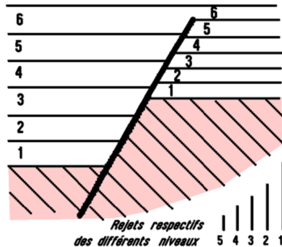
- b - Faille inverse à rejet progressif
