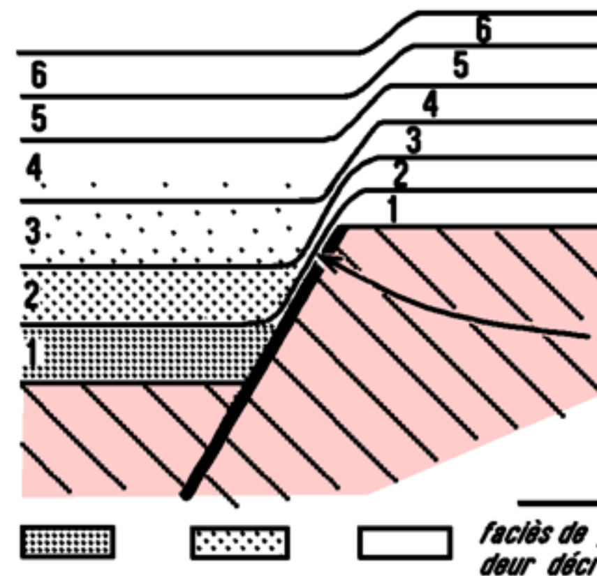
- b - Faille inverse à rejet progressif
